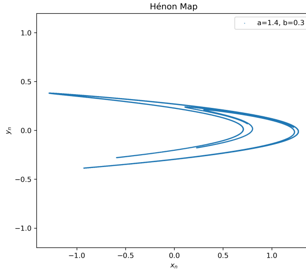
Figure 1: Henon Map 에서 a=1.4 , b=0.3 일때의 그래프를 나타낸다.
