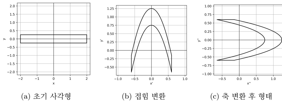
Figure 3: 해논맵에서 사각형 영역이 접히고 수축되는 과정을 나타낸 그림이다.
